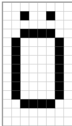
0x99
