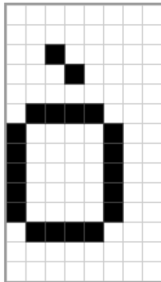
0x95
