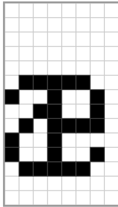
0x91
