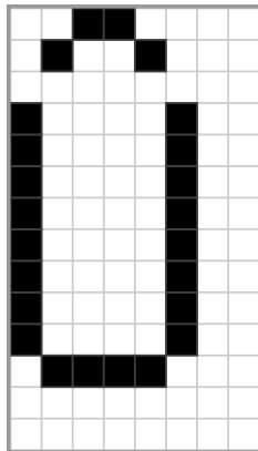
0x9D
